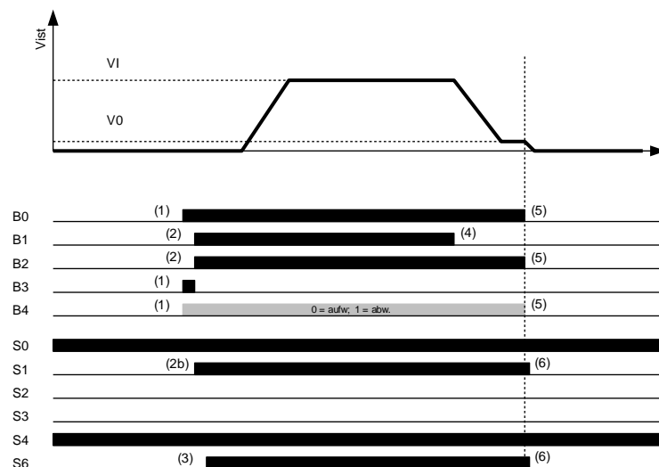
Abbildung 9-3: Inspektionsfahrt
