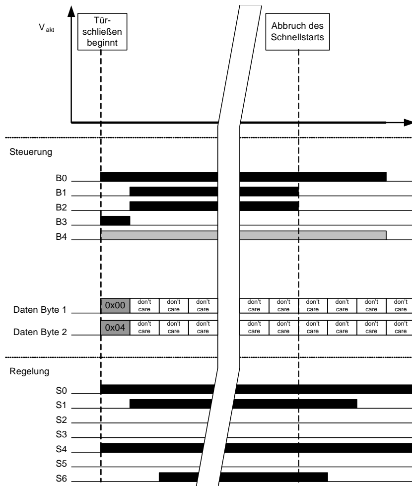
DCP3: kontrolliertes vorzeitiges Beenden des Schnellstarts
