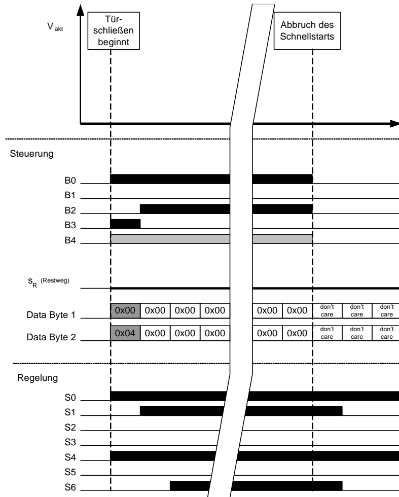
DCP4: Unmittelbarer Abbruch des Schnellstarts
