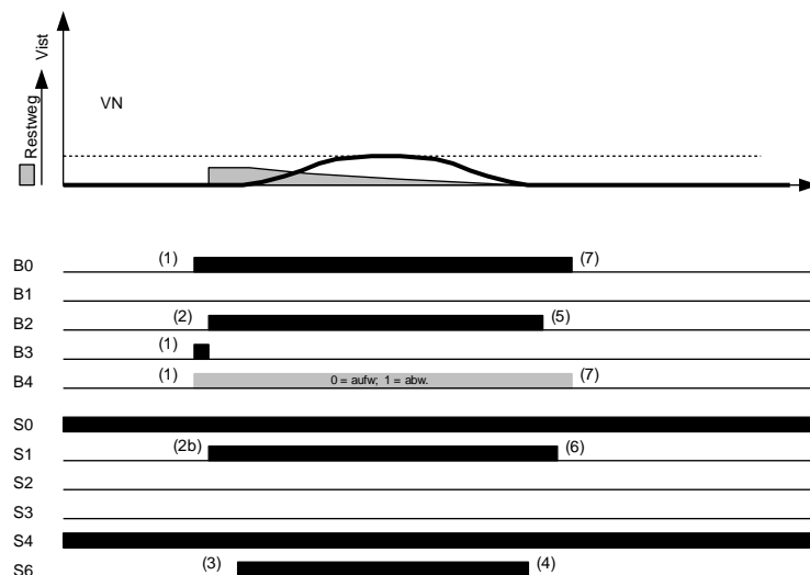
Abbildung 11-7: VN'-Nachstellfahrt (DCP4)
