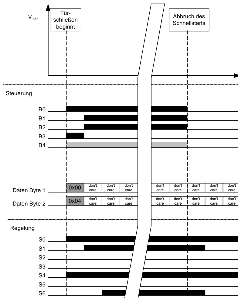
DCP3: Unmittelbarer Abbruch des Schnellstarts
