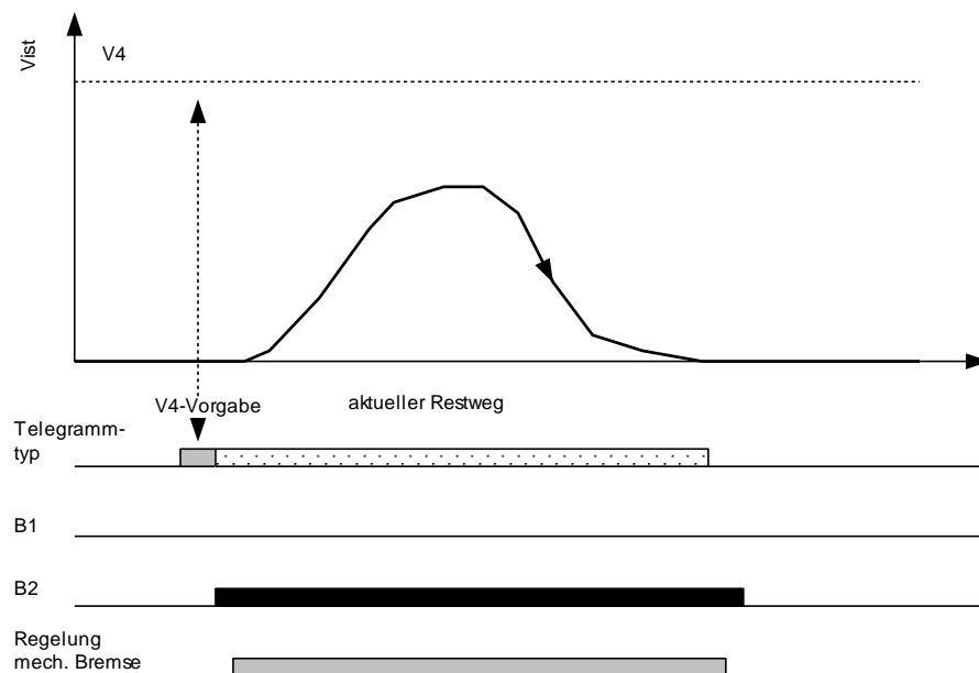
Abbildung 11-2: Restwegorientierte Fahrt (DCP4)
