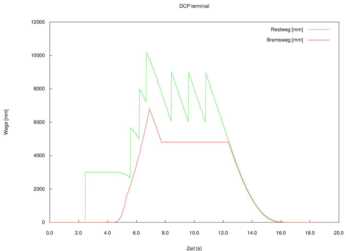
Abbildung 11-1: Restwegorientierte Fahrt mit aktuellem Bremsweg (DCP4)
