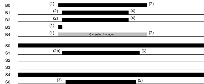
DCP3-Fahrt mit V0
