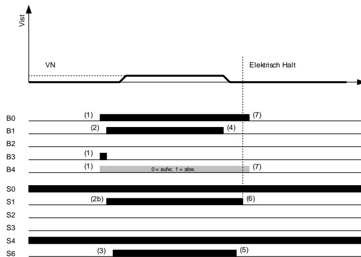
Abbildung 9-6:Nachstellfahrt mit elektr. Halt (DCP3)
