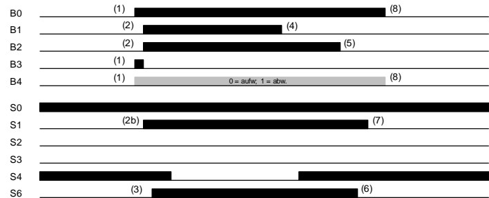
DCP3-Fahrt mit V4
