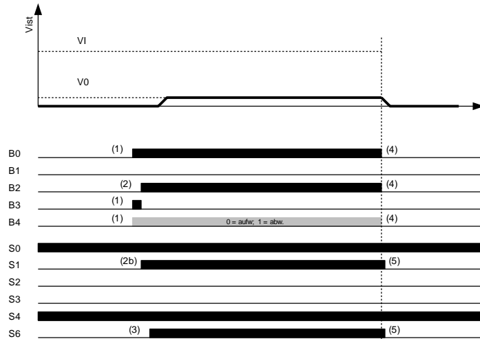
Inspektionsfahrt mit V0 (DCP3 und DCP4)
