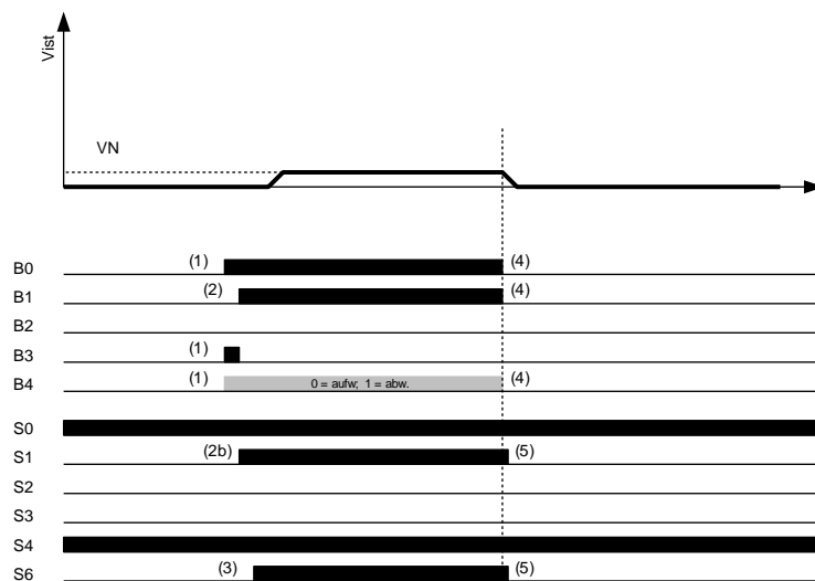
Abbildung 9-5: Nachstellfahrt ohne elektr. Halt (DCP3)
