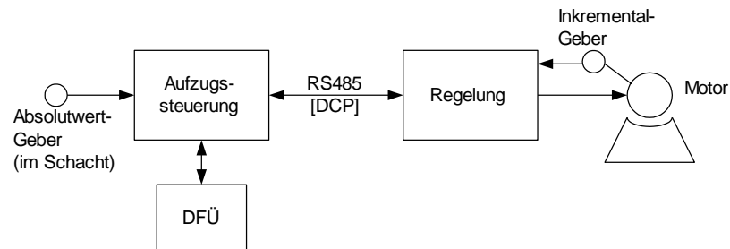
Abbildung 2-1: Regelanbindung über DCP
