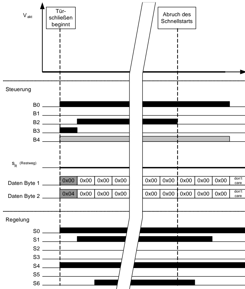
DCP4: kontrolliertes vorzeitiges Beenden des Schnellstarts
