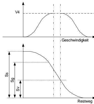
Abbildung 11-6: Fernfahrt
