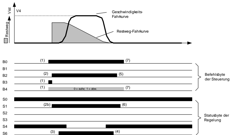
Abbildung 8-1: Diagrammaufbau
