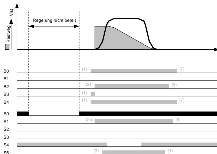
Abbildung 9-1: "Regelung-Bereit"-Bit
