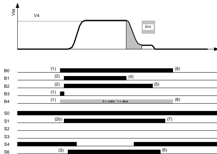
Abbildung 10-1: V4-Fernfahrt (DCP3)
