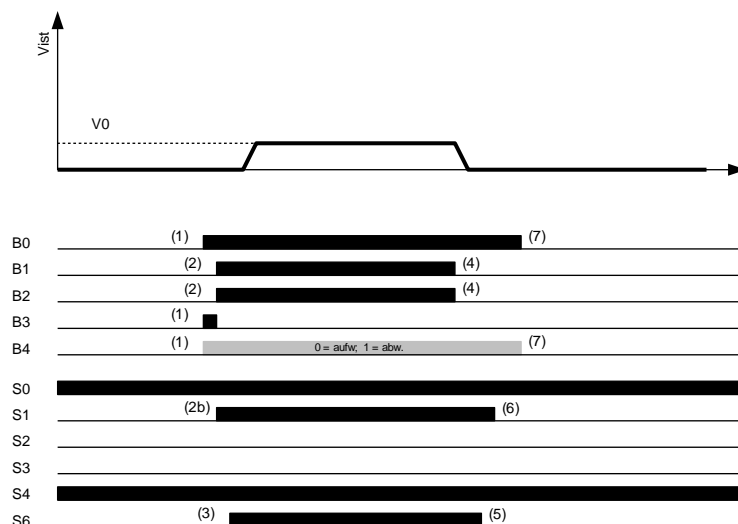
Abbildung 10-3: Schleichfahrt (DCP3)
