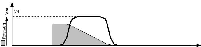
DCP3-Fahrt mit V4
