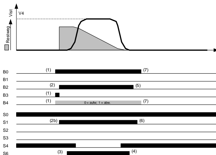
Abbildung 11-3: V4'-Fernfahrt (DCP4)
