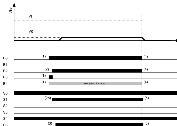
Abbildung 9-4: Inspektionsfahrt mit V0
