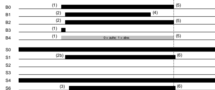
Inspektionsfahrt mit V1 (DCP3 und DCP4)
