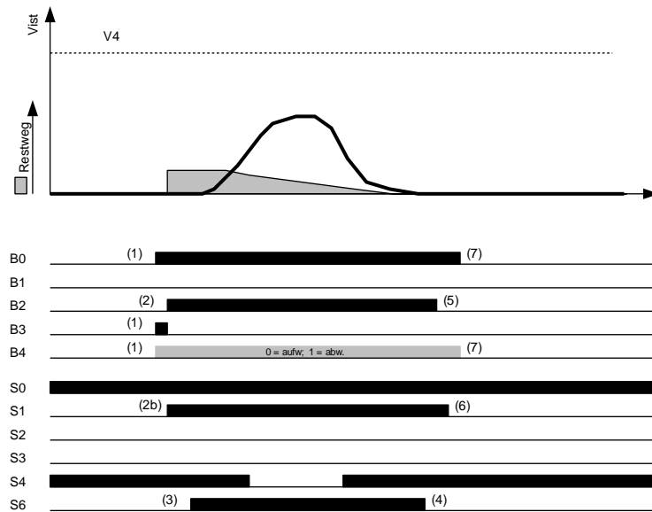
Abbildung 11-4: V4'-Kurzfahrt (DCP4)
