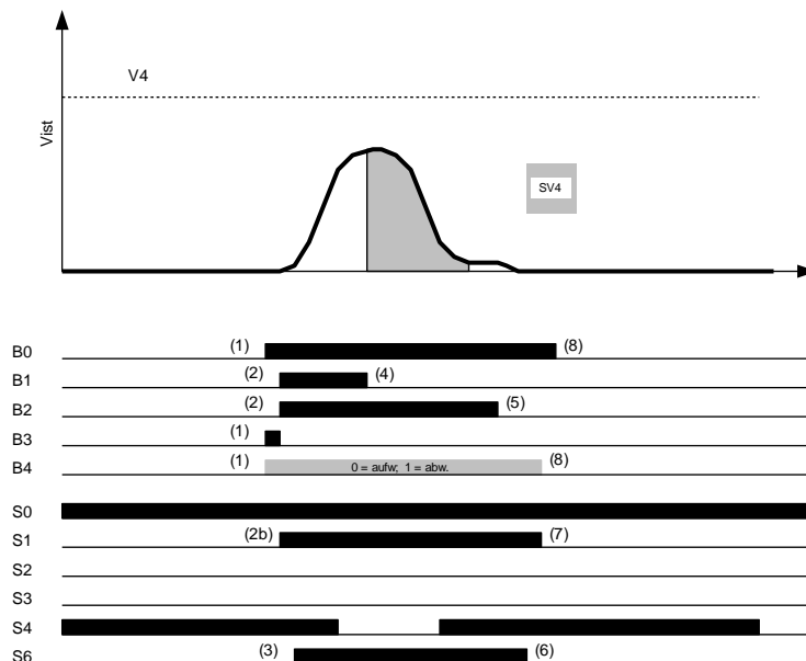
Abbildung 10-2: V4-Kurzfahrt (DCP3)
