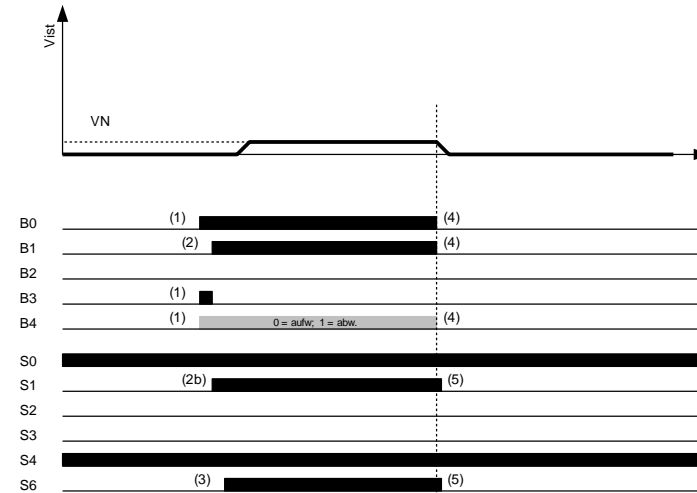
DCP3-Fahrt mit VN ohne "elektrisch Halt"
