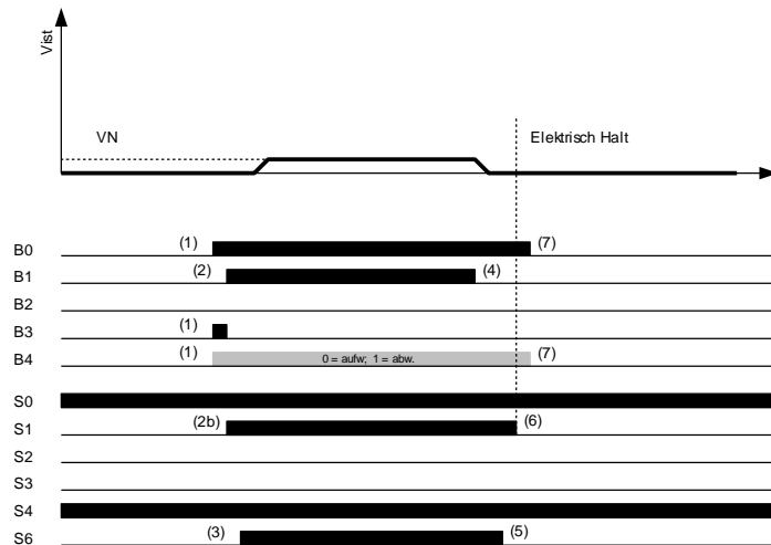
DCP3-Fahrt mit VN mit "elektrisch Halt"
