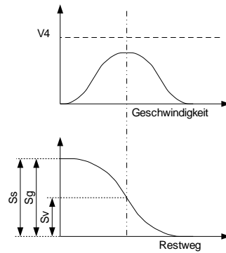
Abbildung 11-5: Kurzfahrt
