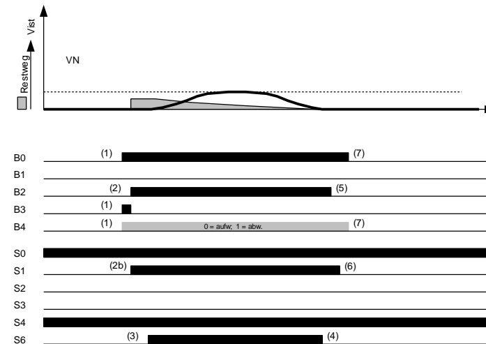
DCP4-Fahrt mit VN
